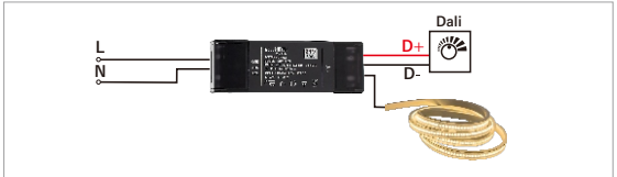
Dali调光【连接示意图】 Dali Dimmer Connection diagram
