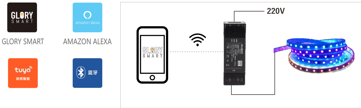
【连接示意图】 Connection diagram
